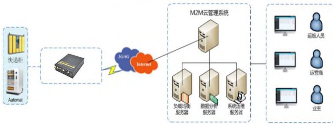
厦门四信设备云管理系统应用拓扑图
